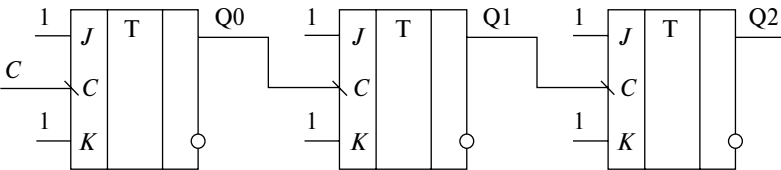
Рис. 2.51. Схема асинхронного трехразрядного счетчика
