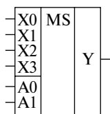
Рис. 2.30. Обозначение мультиплексора на принципиальных схемах
