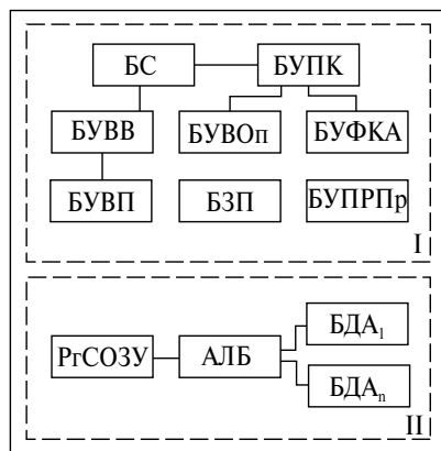
Рис. 1.8. Общая логическая структура микропроцессора:
