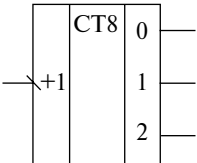
Рис. 2.52. Условно-графическое обозначение трехразрядного суммирующего счетчика
