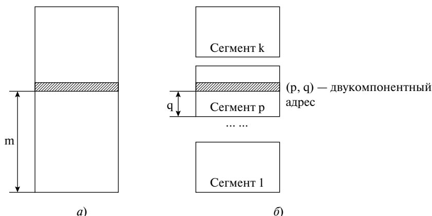
Рис. 5.7. Типы виртуальных адресных пространств: а — плоское, б — сегментированное
