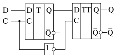
Рис. 2.49. Схема универсального D-триггера
