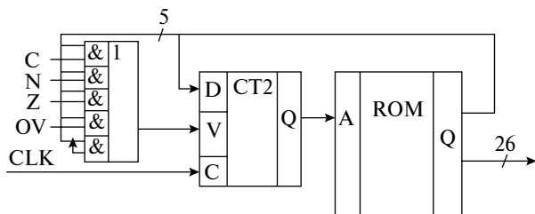
Рис. 3.6. Блок микропрограммного управления микропроцессора
