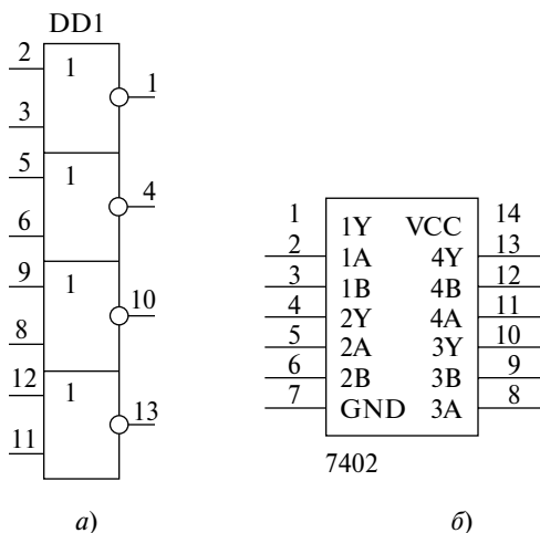
Рис. 2.3. Четыре логических элемента «2ИЛИ-НЕ»: а — микросхема КР1533ЛЕ 1; б — аналог SN74ALS02
