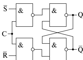
Рис. 2.44. Схема синхронного триггера на схемах «И»
