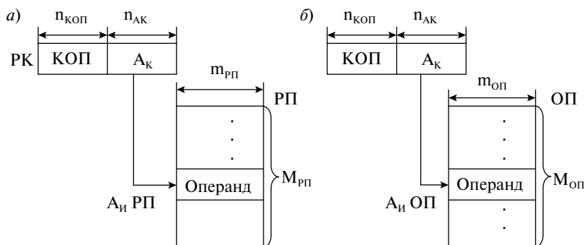
Рис. 4.14. Схема прямой адресации: а — к регистровой памяти; б — к основной памяти
