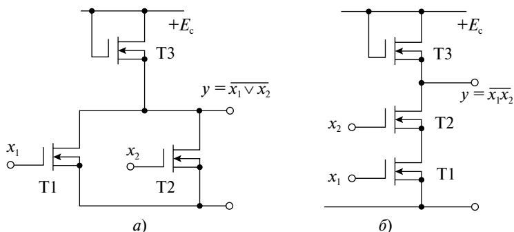
Рис. 2.13. Логические элементы на МОП-транзисторах: а — элемент «ИЛИ-НЕ»; б — элемент «И-НЕ»
