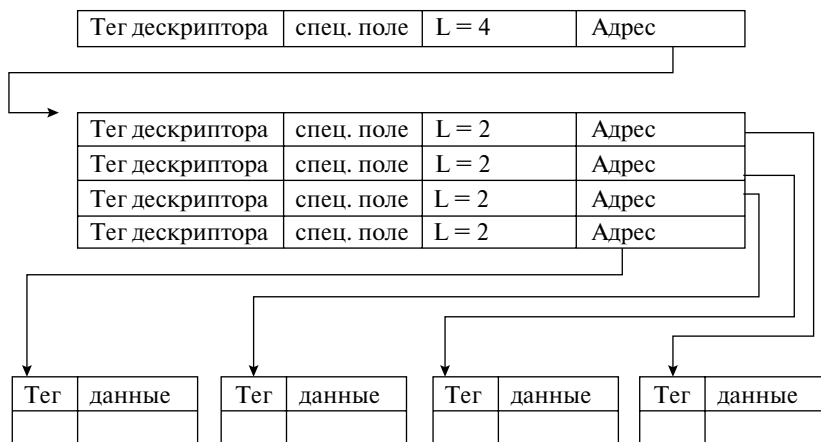
Рис. 4.17. Описание двухмерного массива
