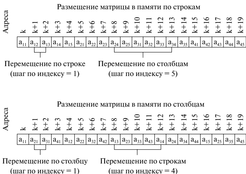
Рис. 7.2. Способы размещения в памяти матрицы 4 \times 5
