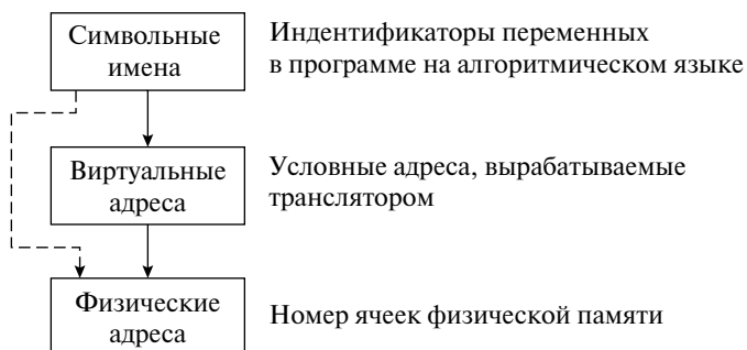
Рис. 5.4. Идентификация переменных и команд
