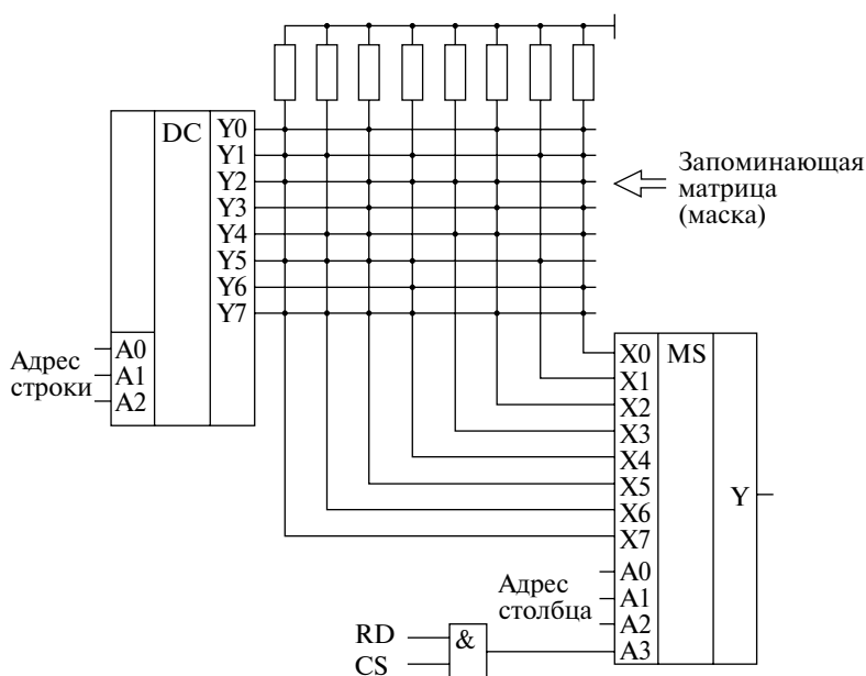
Рис. 2.63. Схема масочного ПЗУ
