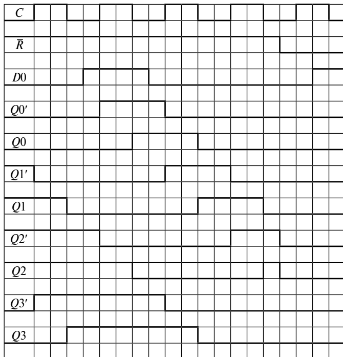
Рис. 2.59. Временная диаграмма работы регистра сдвига
