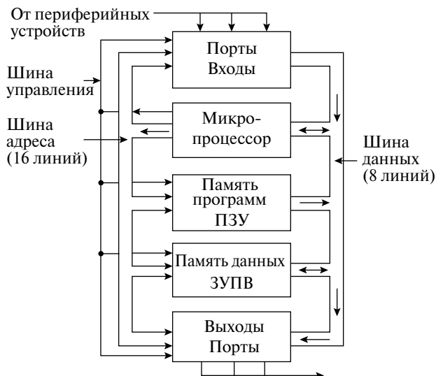
Рис. 1.6. Архитектура типового микропроцессора
