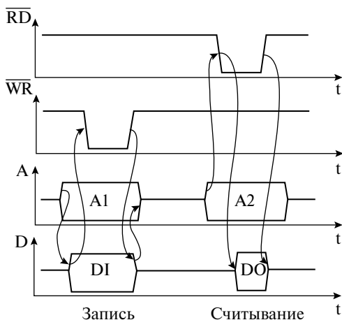
Рис. 3.8. Временные диаграммы считывания команды микропроцессором
