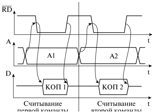
Рис. 3.9. Временные диаграммы сигналов считывания команд из ОЗУ
