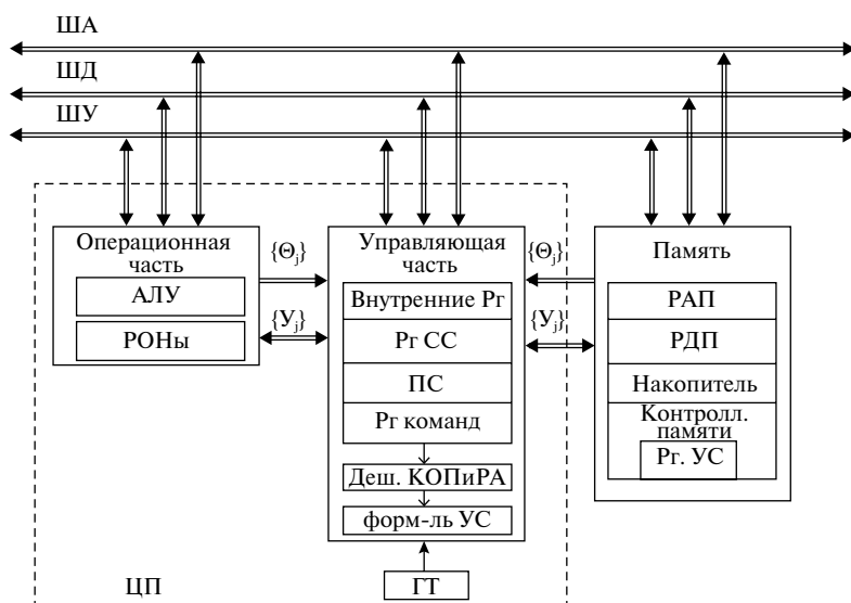
Рис. 4.18. Типовая структура процессора и основной памяти
