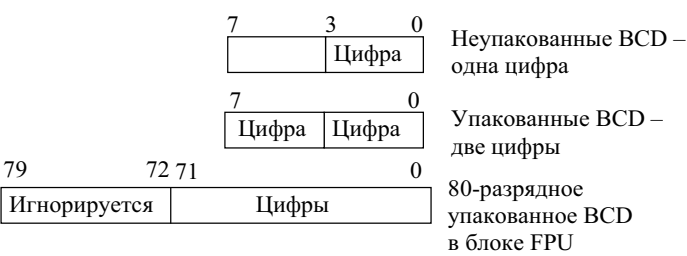
Рис. 4.3. Форматы двоично-десятичных данных
