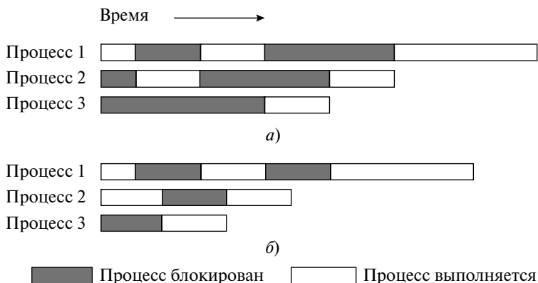
Рис. 7.7. Мультипрограммирование и мультипроцессорная обработка: а — мультипрограммирование; б — мультипроцессорная обработка
