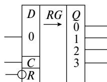
Рис. 2.58. Условно-графическое обозначение четырехразрядного регистра сдвига с асинхронным входом установки в «0»
