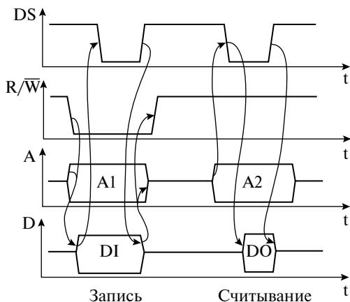
Рис. 2.74. Временная диаграмма обращения к ОЗУ, принятая для схем, совместимых со стандартом фирмы «Motorola»
