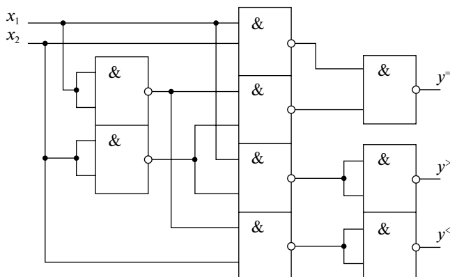
Рис. 2.25. Одноразрядный компаратор двоичных чисел
