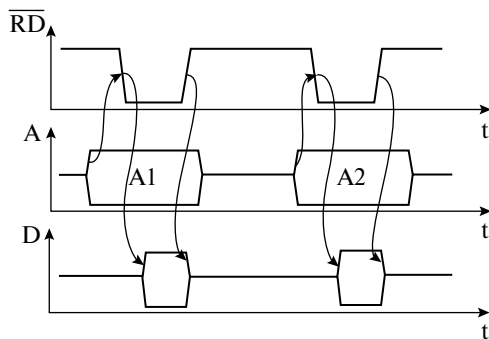
Рис. 2.69. Временная диаграмма чтения информации из ПЗУ
