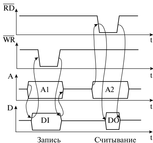
Рис. 2.73. Временная диаграмма обращения к ОЗУ, принятая для схем, совместимых со стандартом фирмы «Intel»
