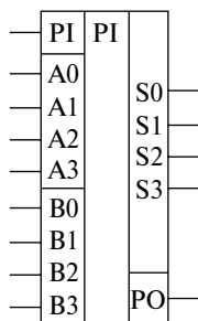
Рис. 2.24. Изображение полного двоичного многоразрядного сумматора на схемах
