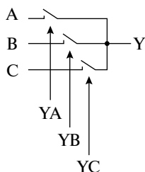
Рис. 2.26. Коммутатор (мультиплексор), собранный на ключах
