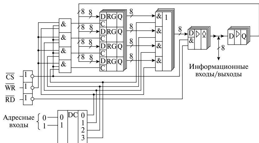
Рис. 2.70. Структурная схема ОЗУ
