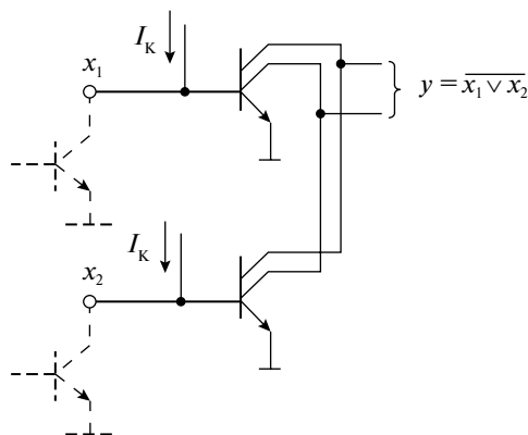
Рис. 2.12. Реализация схемы «ИЛИ-НЕ» в логике И 2 Л
