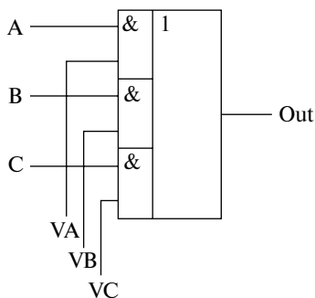
Рис. 2.28. Схема мультиплексора на логических элементах
