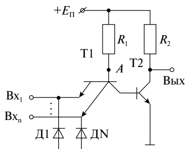
Рис. 2.10. Базовый элемент ТТЛ
