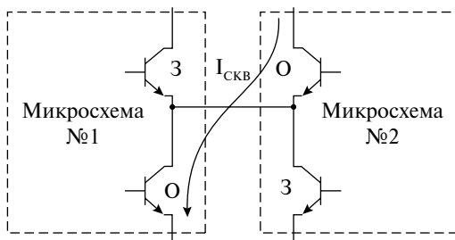
Рис. 2.37. Путь протекания сквозного тока при непосредственном соединении выходов цифровых микросхем
