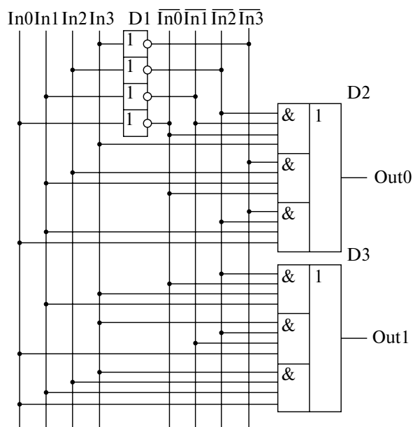
Рис. 2.6. Принципиальная схема, реализующая таблицу истинности, приведенную на рис. 2.5
