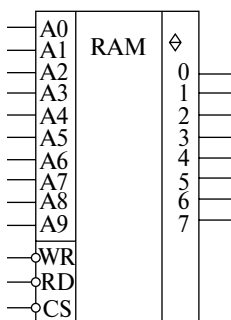
Рис. 2.71. Изображение ОЗУ на принципиальных схемах
