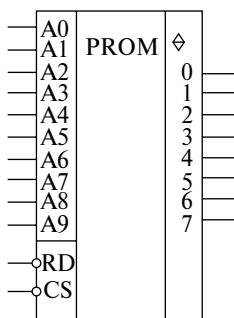
Рис. 2.65. Обозначение программируемого ПЗУ на принципиальных схемах
