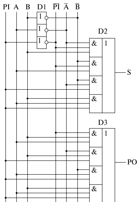
Рис. 2.21. Принципиальная схема, реализующая таблицу истинности полного двоичного одноразрядного сумматора
