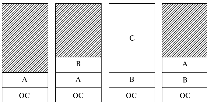
Рис. 5.3. Свопинг (подкачка) — процесс целиком загружается в память
