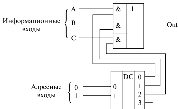
Рис. 2.29. Принципиальная схема мультиплексора, управляемого двоичным кодом
