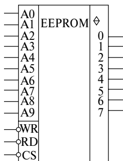
Рис. 2.67. Обозначение электрически стираемого ПЗУ на принципиальных схемах
