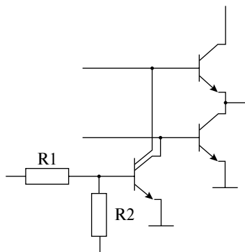
Рис. 2.38. Принципиальная схема выходного каскада микросхемы с тремя состояниями на выходе
