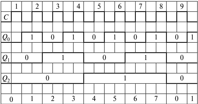
Рис. 2.53. Временная диаграмма работы счетчика
