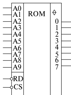
Рис. 2.64. Обозначение масочного ПЗУ на принципиальных схемах
