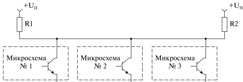
Рис. 2.34. Схема монтажного «ИЛИ»
