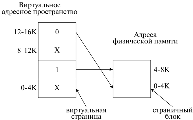
Рис. 5.5. Страничная организация памяти
