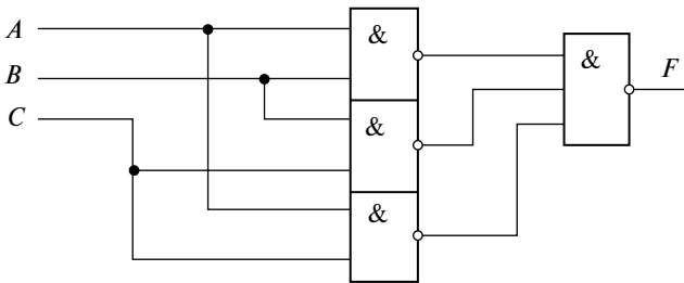
Рис. 2.7. Реализация функции F = AB \vee BC \vee AC в базисе «И-НЕ»
