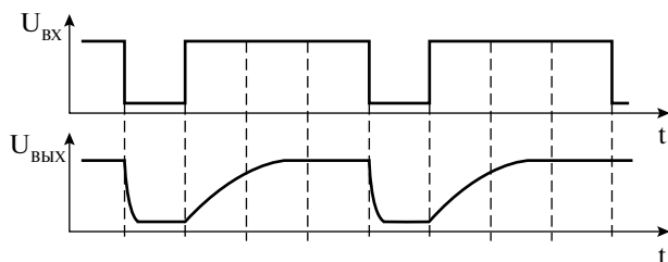
Рис. 2.36. Временные диаграммы напряжения на входе и выходе микросхемы с открытым коллектором
