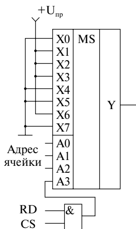
Рис. 2.60. Схема ПЗУ, построенная на мультиплексоре
