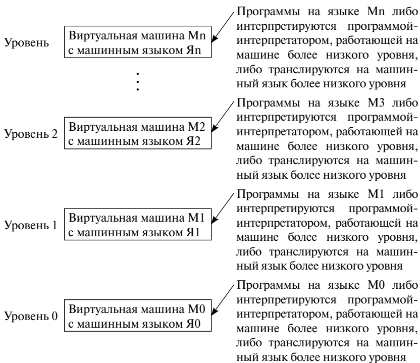
Рис. 1.1. Структура многоуровневой вычислительной машины
