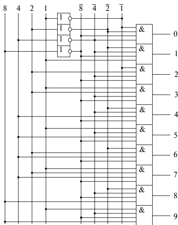
Рис. 2.33. Принципиальная схема двоично-десятичного декодера
