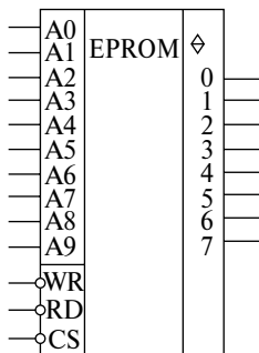
Рис. 2.66. Обозначение репрограммируемого ПЗУ на принципиальных схемах
