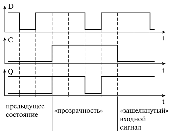
Рис. 2.48. Временная диаграмма D триггера (зашелки)
