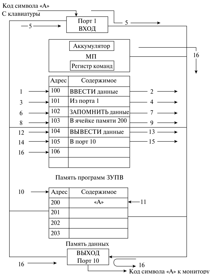
Рис. 1.7. Диаграмма выполнения процедуры ввода-запоминания-вывода
