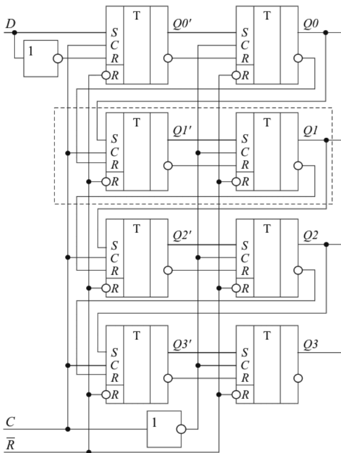
Рис. 2.57. Структура регистра сдвига
