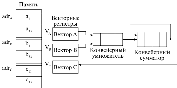
Рис. 7.4. Векторный процессор для вычисления скалярного произведения
