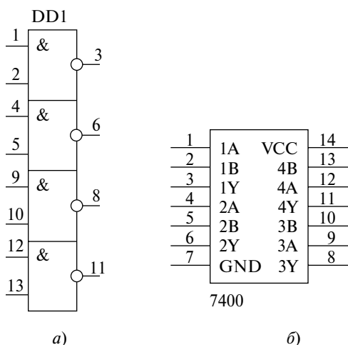
Рис. 2.2. Четыре логических элемента «2И-НЕ»: а — микросхема КР1533ЛА3; б — аналог SN74ALS00A
