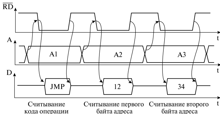
Рис. 3.10. Временная диаграмма выполнения команды JMP 1234
