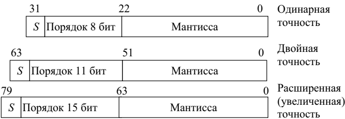
Рис. 4.2. Форматы данных с плавающей точкой
