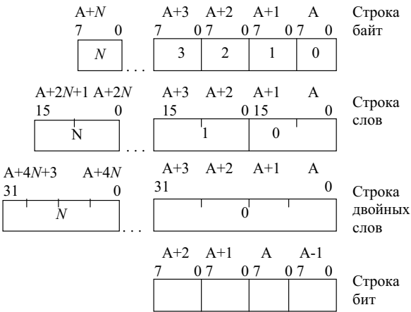
Рис. 4.4. Данные типа «строка»
