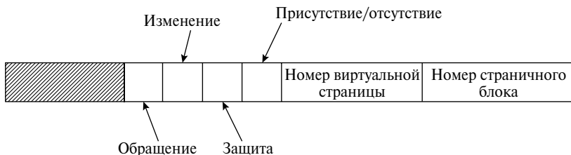
Рис. 5.6. Типичная запись в таблице страниц
