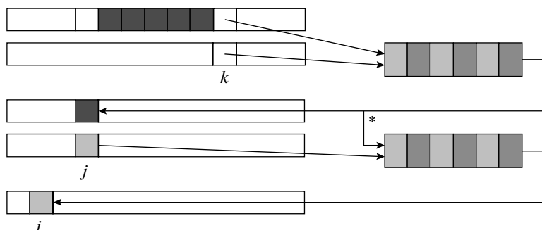
Рис. 7.6. Сцепление векторов
