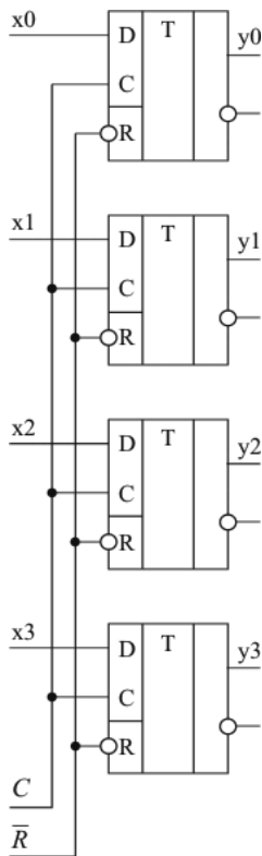
Рис. 2.55. Структура четырехразрядного регистра хранения с асинхронным входом установки в «0»
