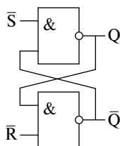
Рис. 2.41. Схема простейшего триггера на схемах «И»
