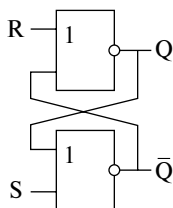
Рис. 2.42. Схема простейшего триггера на схемах «ИЛИ».
