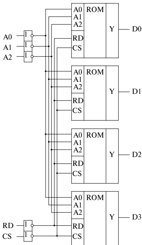
Рис. 2.62. Схема многоразрядного ПЗУ
