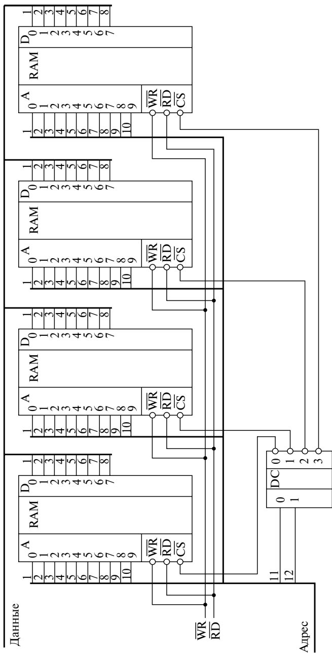
Рис. 2.72. Схема ОЗУ, построенного на нескольких микросхемах памяти
