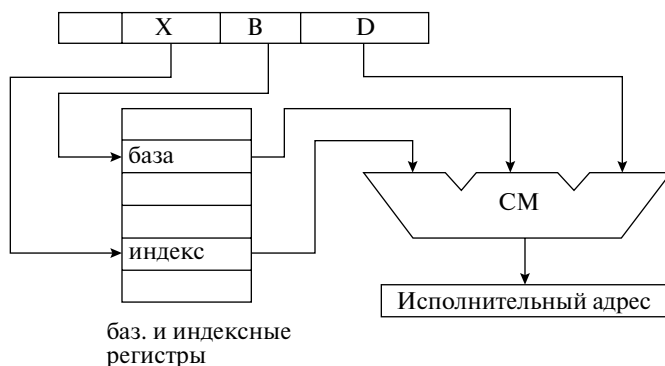
Рис. 4.16. Формирование исполнительного адреса операнда при индексации
