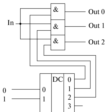
Рис. 2.31. Принципиальная схема демультиплексора, управляемого двоичным кодом
