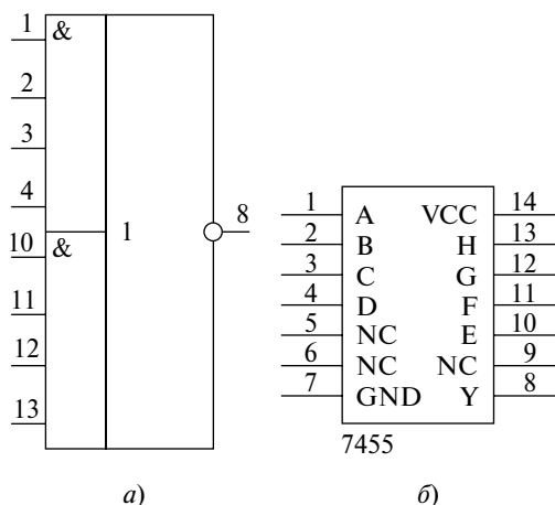
Рис. 2.4. Логический элемент «2-4И-2ИЛИ-НЕ»: а — микросхема К555ЛР4, б — аналог SN74LS55
