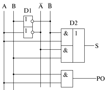
Рис. 2.18. Принципиальная схема, реализующая таблицу истинности полусумматора
