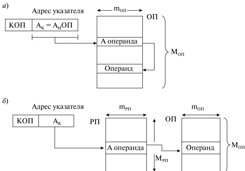
Рис. 4.15. Схема косвенной адресации:
