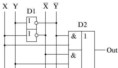
Рис. 2.15. Принципиальная схема, реализующая таблицу истинности сумматора по модулю два
