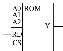
Рис. 2.61. Обозначение ПЗУ на принципиальных схемах
