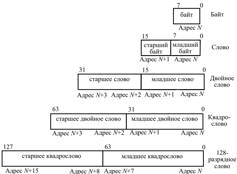
Рис. 4.1. Основные типы данных
