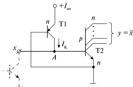
Рис. 2.11. Базовый элемент инжекционной логики
