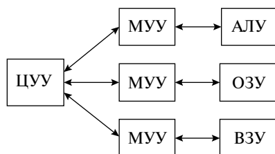
Рис. 3.2. Обобщенная структура УУ
