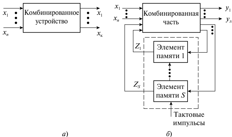
Рис. 2.9. Структура цифрового устройства: а — комбинационного; б — последовательностного
