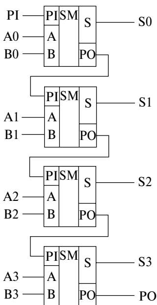
Рис. 2.23. Принципиальная схема многоразрядного двоичного сумматора
