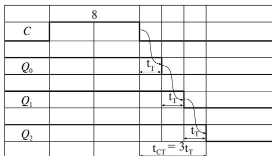
Рис. 2.54. Оценка быстродействия асинхронного счетчика
