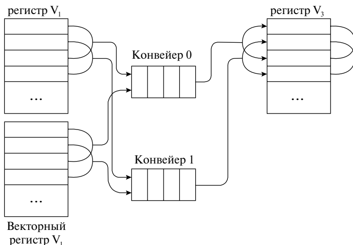
Рис. 7.5. Выполнение векторных операций при двух конвейерах
