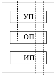
Рис. 1.5. Логические структуры многокристалльного секционного МП
