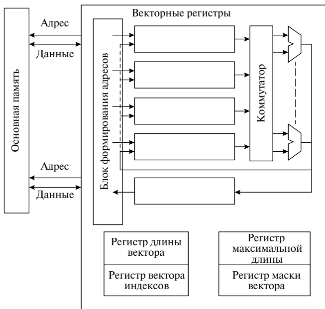
Рис. 7.3. Упрощенная структура векторного процессора
